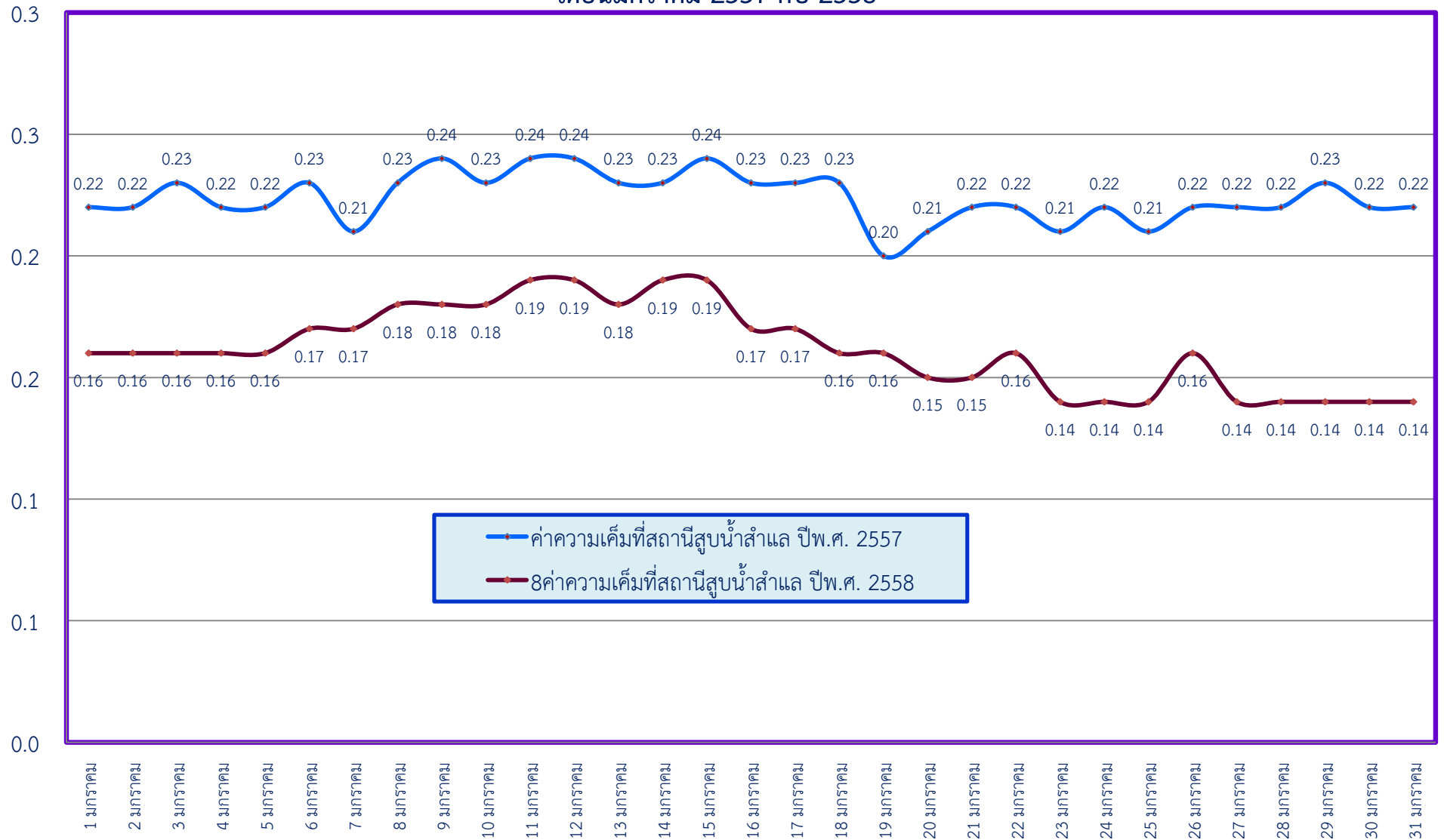
กราฟแสดงการเปรียบเทียบค่าความเค็มในแม่น้ำเจ้าพระยา ที่จุดตรวจวัดทำนายนนท์ จ.นนทบุรี เดือนมกราคม 2557 กับ 2558
